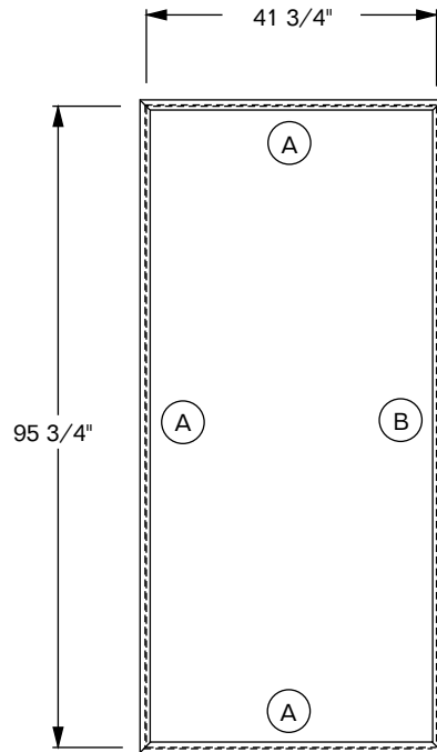
MODEL 1404-6822-L THERMAL DOOR GASKET INNER, LEFT
