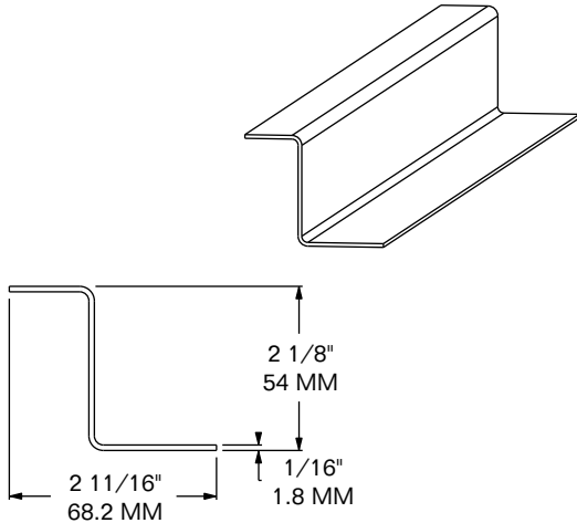
MODEL 1405-7439 DOOR STRINGER
